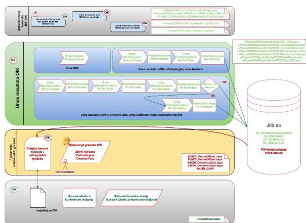
Slika 7. Dijagram funkcionalnih cjelina novog modula
